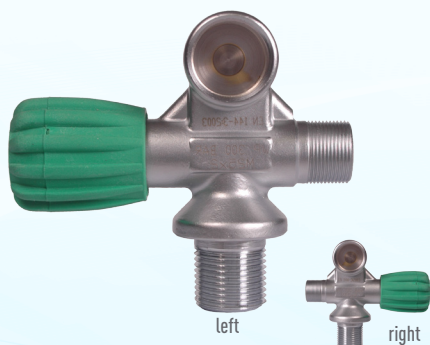
Modu valve M26 300 BAR M25x2 #N10155SD3 left #N10156DD3 right
